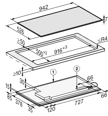
KM 7899 FL installazione a filo
