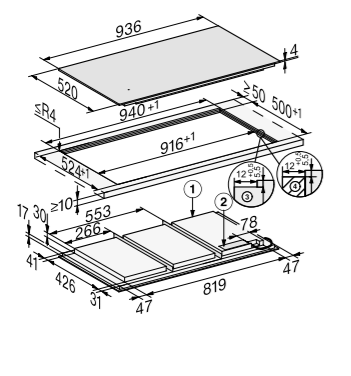
KM 7897 FL installazione a filo
