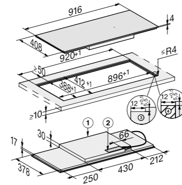
KM 7999 FL installazione a filo
