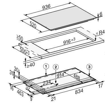
KM 7999 FL installazione in appoggio
