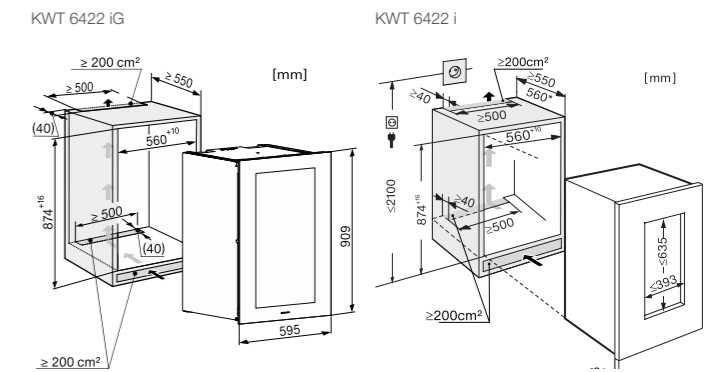
Schemi per KWT 6422 iG
