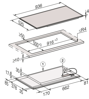
KM 7594 FL installazione in appoggio
