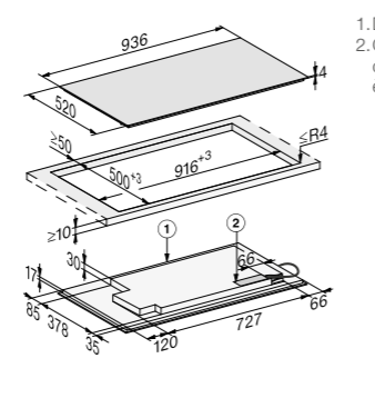
KM 7897 FL installazione in appoggio
