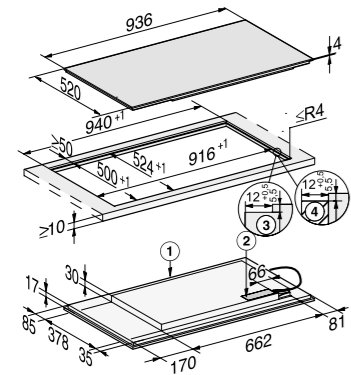
KM 7699 FR installazione in appoggio
